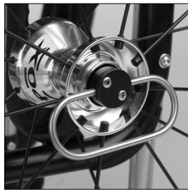
MG 28 Tetraentriegelung
